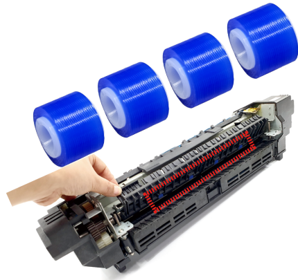
[Xr-C12] 固定徽章滚轮 定影单元进纸部发生卡纸时需要更换的滚轮。该滚轮坚固耐用，使用寿命长。
