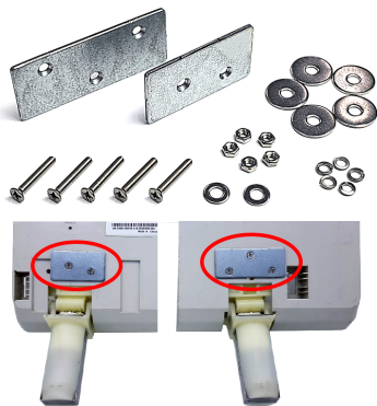
[Xi-001] 平衡支撑轴改进 当支撑复印机 RADF 的平衡固定部件损坏时可以轻松更换的产品。
